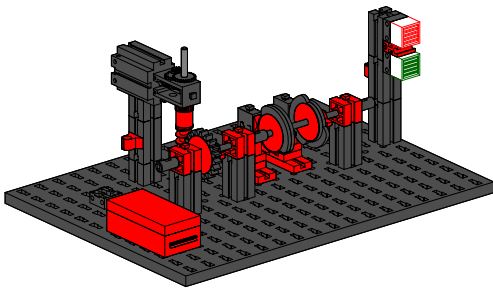
Ampelsteuerung / Traffic light control / Commande des feux de signalisation / Regeling van een verkeerslicht / Mando del semáforo / Comando de semáforo
