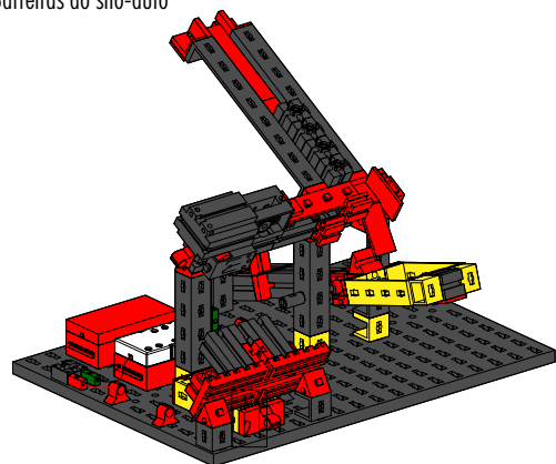
Bausteinspender / Brick dispenser / Distributeur d'éléments de construction / Bouwsteenautomaat / Dispensador de elementos / Distribuidor do componente
